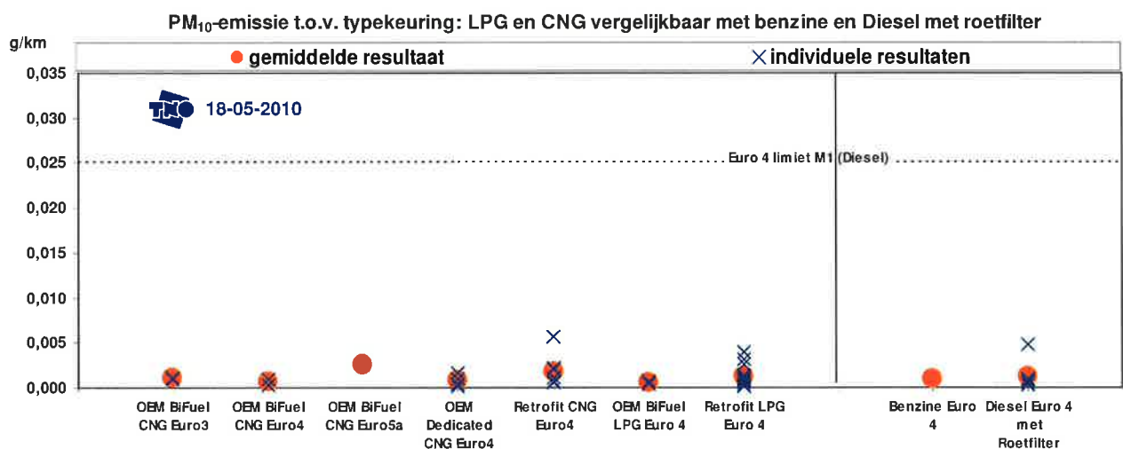
Figuur 8: \text{PM}_{10} -emissie tijdens de typekeurtest in vergelijking met Euro-4 benzine- en diesellovoertuigen met roetfilter
